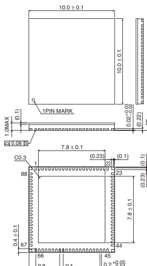
UQFN88MV0100
