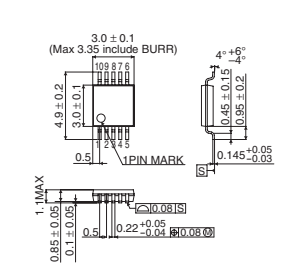
TSSOP-C10J
