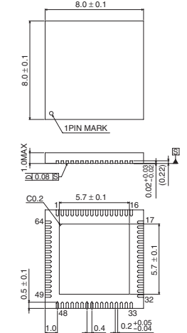
UQFN064V8080
