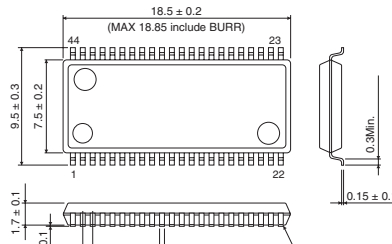
SSOP-A44
