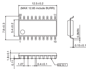
SOP20
