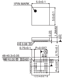
VBGA131T070
