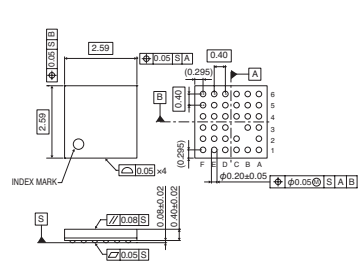
WL-CSP34
