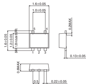
VSO5
