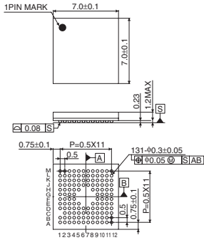
VBGA131T070
