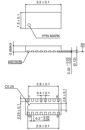
USON016X3315
