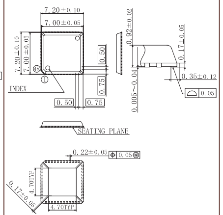
VQFN48
