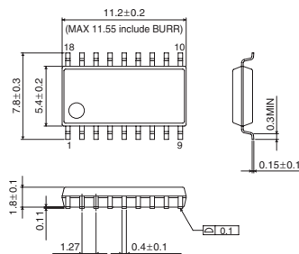
SOP18
