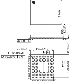
VBGA161T080
