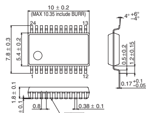
SSOP-A24
