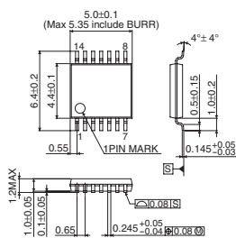
TSSOP-B14J
