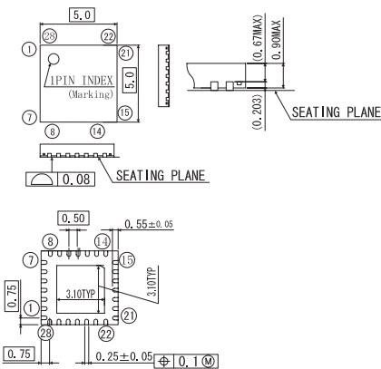
VQFN28
