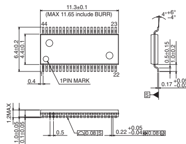
TSSOP-C44
