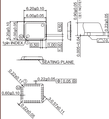
VQFN32
