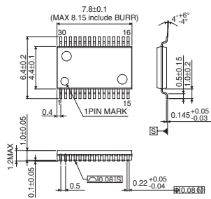
TSSOP-C30
