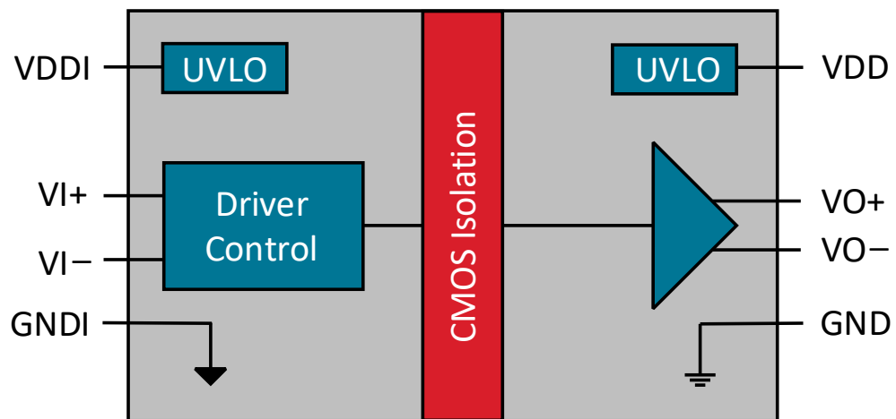
Si82A40x/43x
